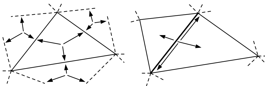
Рис. 8. Связи треугольников (слева) и ребер (справа) структуры “Узлы, ребра и треугольники”
