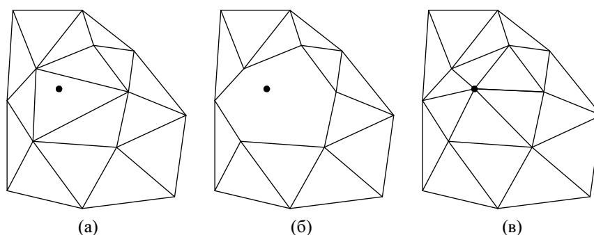
Рис. 14. Вставка точки в итеративном алгоритме “Удаляй и строй”
