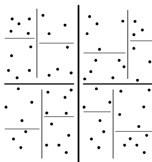
Рис. 22. Разбиение множества точек в алгоритме триангуляции “Раздели и властвуй”
