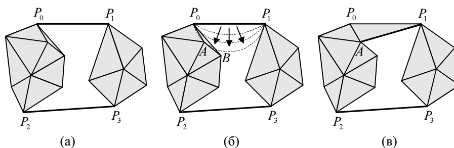
Рис. 24. Слияние триангуляций (а — поиск касательных, б — поиск ближайшего соседа Делоне для базовой линии, в — построение треугольника)
