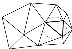
Рис. 1. Триангуляция Делоне
