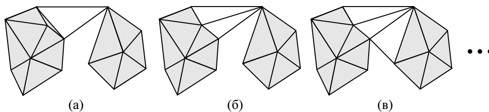
Рис. 26. Шаги слияния “Строй, перестраивая” (а — построение первого треугольника, б — немедленные перестроения, в — построение второго треугольника)
