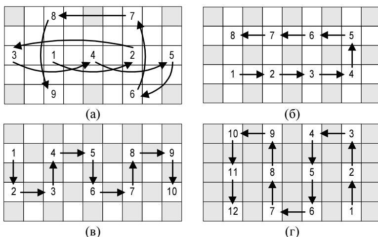
Рис. 18. Порядок выбора точек в итеративном алгоритме с послынным сгущением
