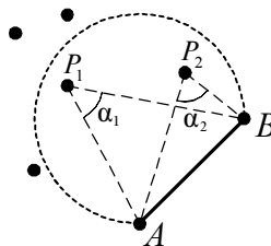
Рис. 31. Выбор очередной точки для включения в триангуляцию
