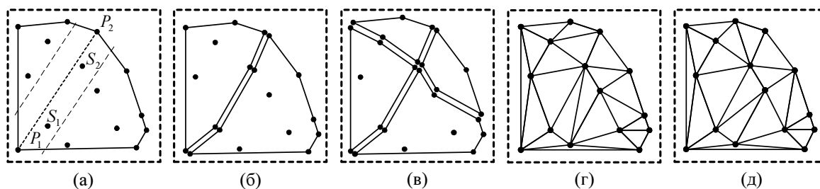
Рис. 37. Алгоритм рекурсивного расщепления (а — выбор направления и коридора, б–г — шаги расщепления, д — перестроение триангуляции)
