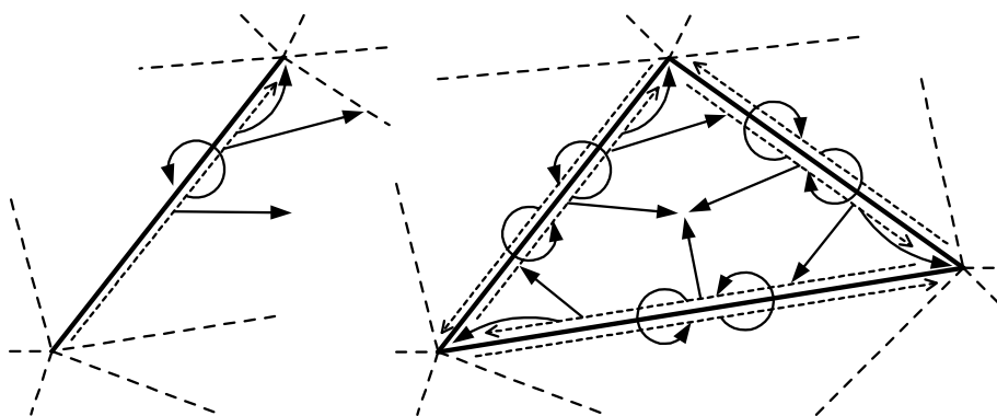
Рис. 6. Связи ребер (слева) и неявное задание треугольников (справа) в структуре “Двойные ребра”
