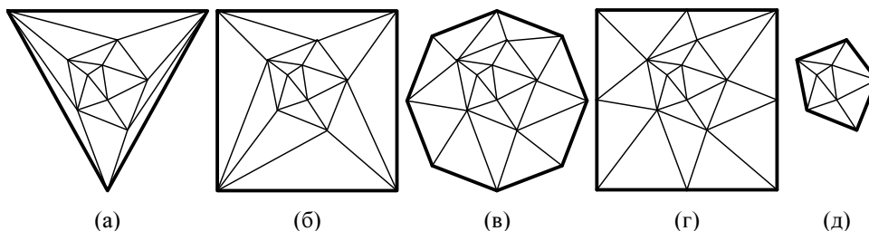
Рис. 12. Варианты суперструктур
