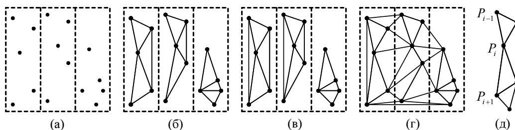
Рис. 29. Алгоритм выпуклого полосового слияния (а-г — шаги работы алгоритма, д — достраивание выпуклости)
